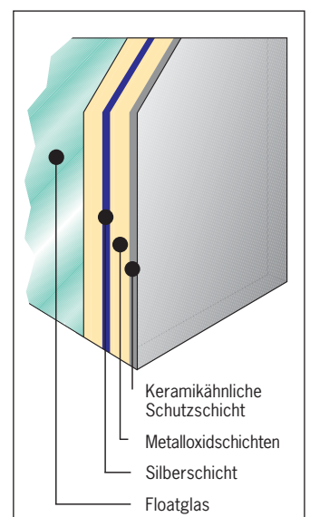
Schematischer Scheibenaufbau von SANCO SILVERSTAR 1.1 Neutral
